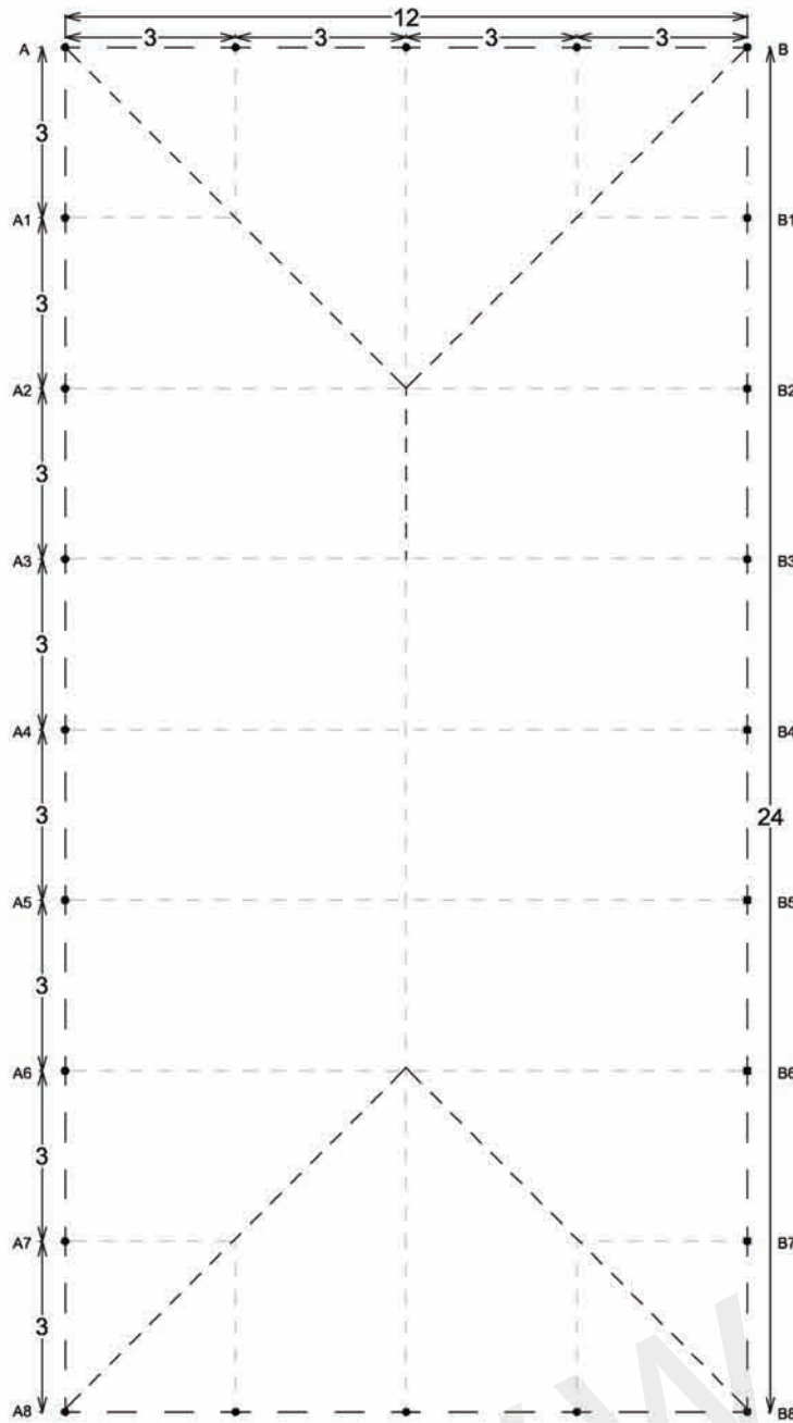
PLANTA
