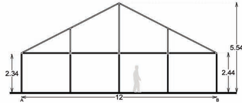
ALZADO 1
