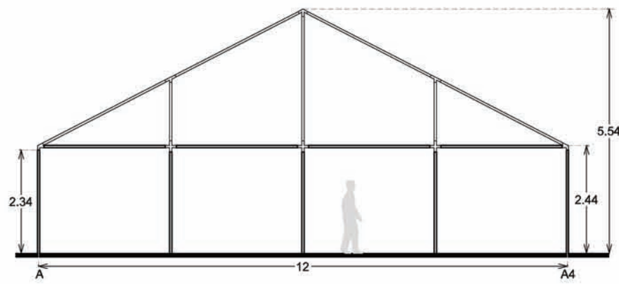
ALZADO 1
