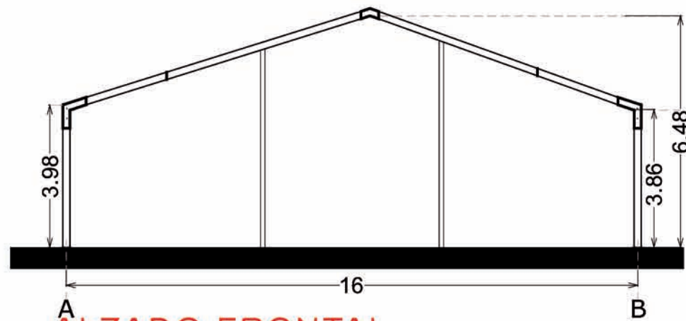
ALZADO FRONTAL
