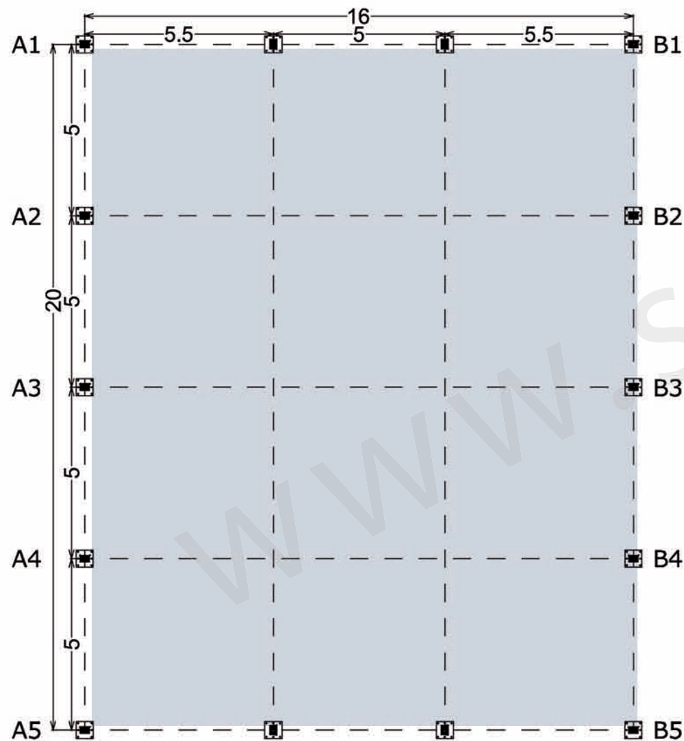
PLANTA
